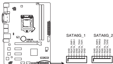
Connecteurs SATA 6.0Gbs de la H81M-PLUS
