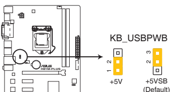
Jumper de mise en route via clavier et USB de la H81M-PLUS
