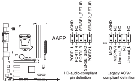
Connecteur audio pour panneau avant de la H81M-PLUS
