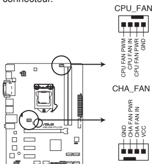
Connecteurs de ventilation de la H81M-PLUS
