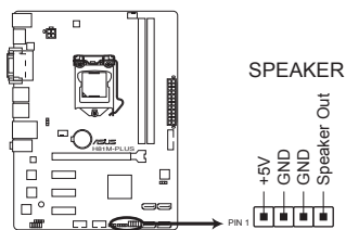
Connecteur pour haut-parleur d'alerte système de la H81M-PLUS
