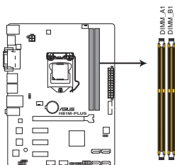
Interfaces de connexion pour modules mémoire DDR3 de la H81M-PLUS
