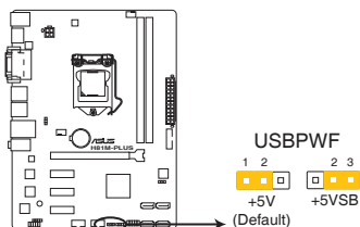
Jumper de mise en route via USB de la H81M-PLUS
