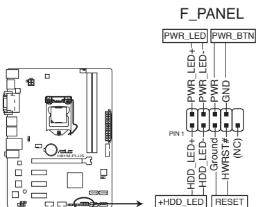
Connecteur panneau système de la H81M-PLUS
