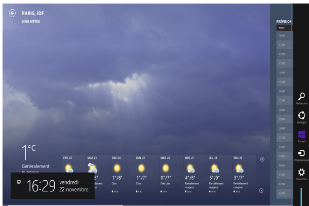
Barre d'action
