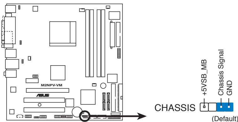
Connecteur Châssis intrusion de la M2NPV-VM
