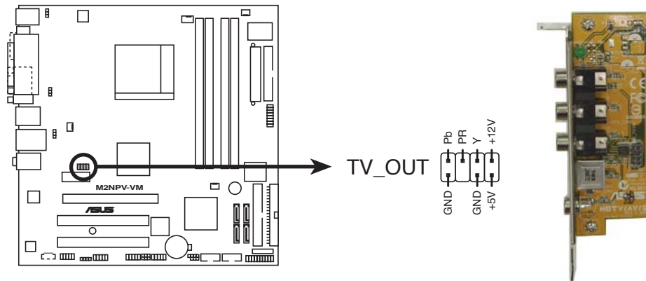
Connecteur TV-Out de la M2NPV-VM
