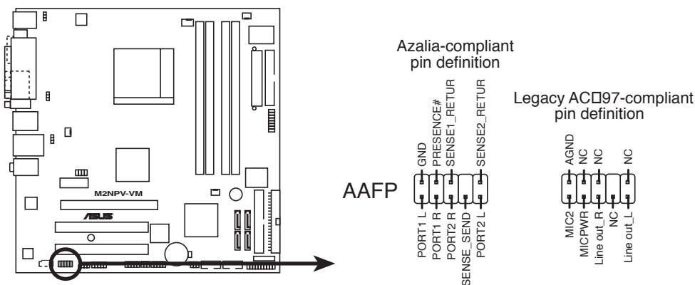
Connecteur Front panel audio de la M2NPV-VM
