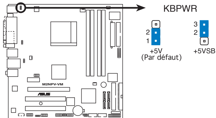
Paramètres d'alimentation du clavier de la M2NPV-VM
