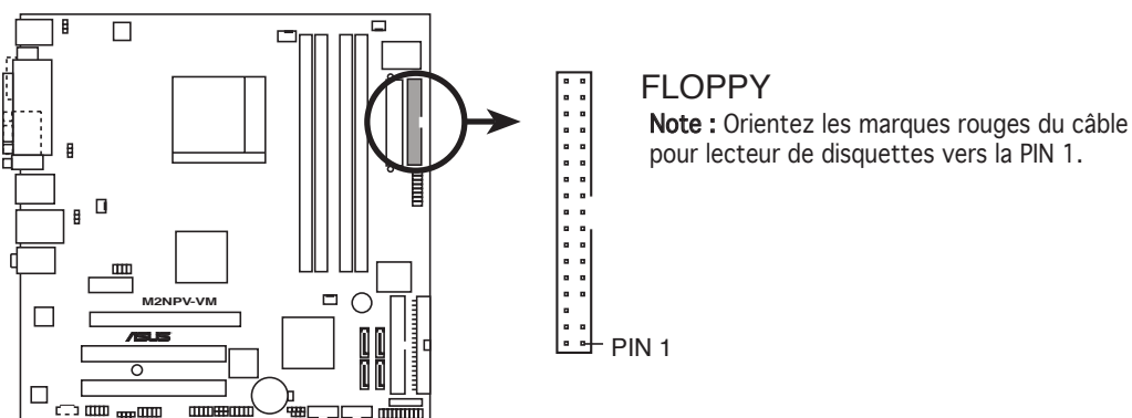
Connecteur lecteur de disquettes de la M2NPV-VM
