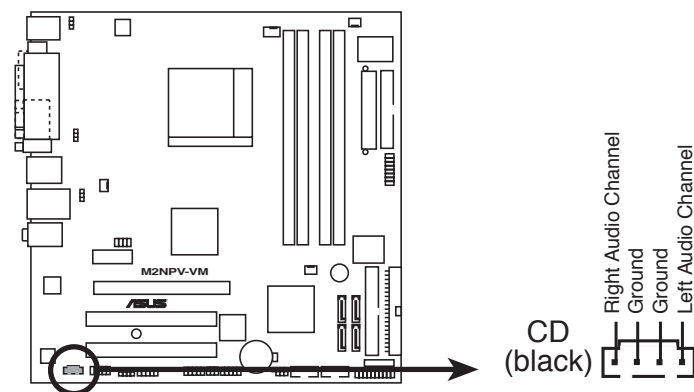
Connecteur audio internes de la M2NPV-VM
