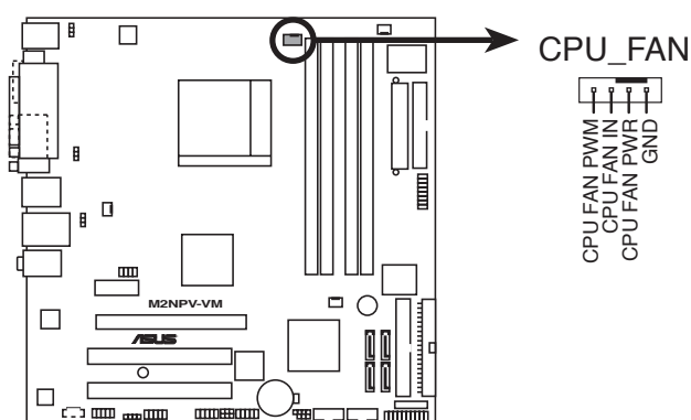
Connecteur CPU_FAN de la M2NPV-VM
