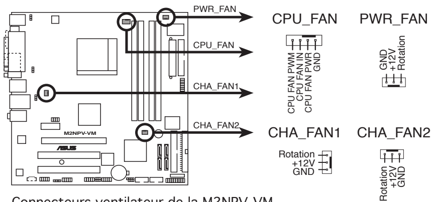
Connecteurs ventilateur de la M2NPV-VM
