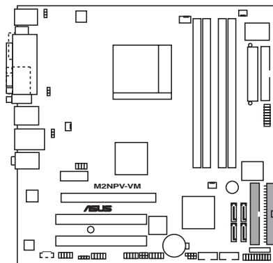
Connecteurs IDE de la M2NPV-VM
