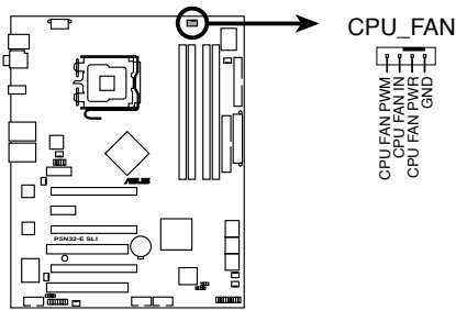
P5N32-E SLI CPU fan connector
