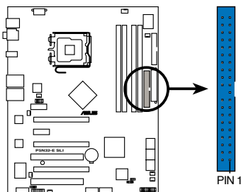
P5N32-E SLI IDE connector
