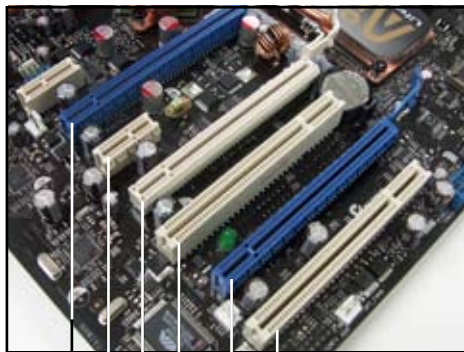
PCI-Steckplatz PCI Express x16-Steckplatz (blau) PCI-Steckplatz PCI Express x16-Steckplatz (x8-Verbindung weiß) PCI Express x1-Steckplatz PCI Express x16-Steckplatz (blau)
