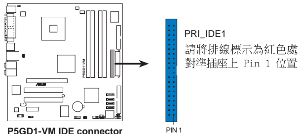
P5GD1-VM IDE connector
