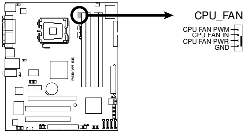
P5B-VM SE CPU Fan Connector
