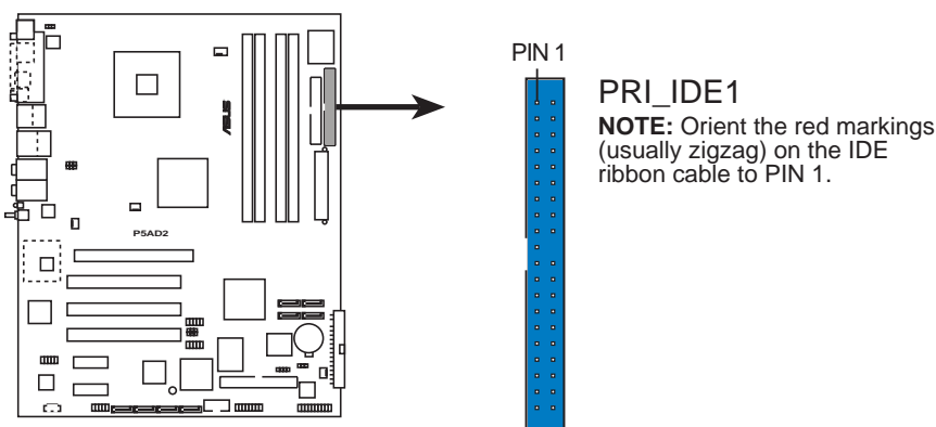
P5AD2 Deluxe IDE connector
