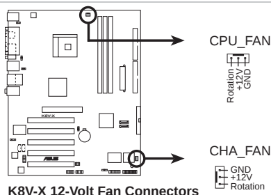
K8V-X 12-Volt Fan Connectors
