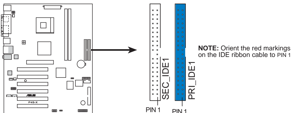
P4S-X IDE Connectors
