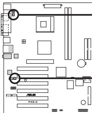
P4S-X 12-Volt Cooling Fan Power
