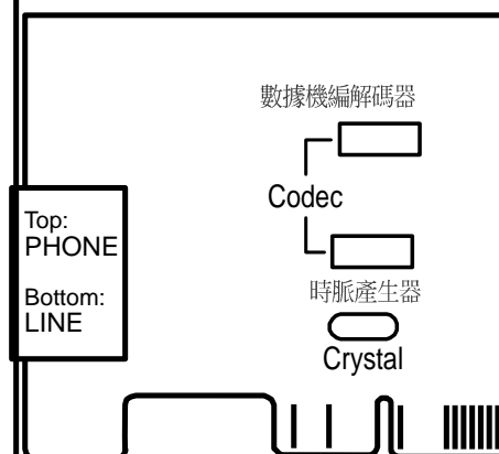
數據機子卡構造圖
