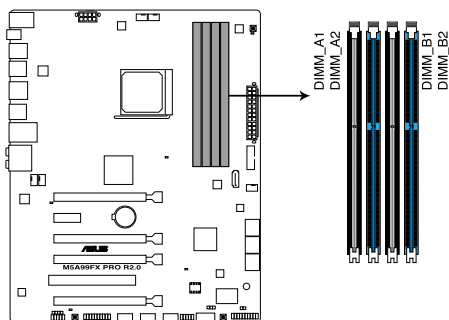
M5A99FX PRO R2.0 240ピン DDR3 DIMM Slots
