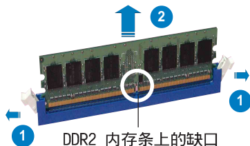
DDR2 内存条上的缺口
