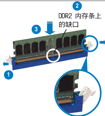
往外扳开内存条插槽两端的白色卡榫
