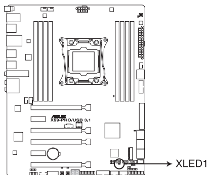
Témoin EZ XMP de la X99-PRO / USB 3.1
