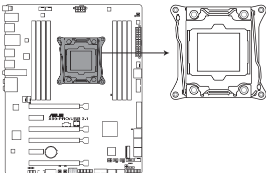
Interface de connexion LGA2011-v3 de la X99-PRO / USB 3.1
