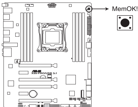
Bouton MemOK! de la X99-PRO / USB 3.1
