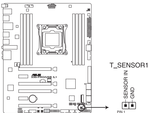
Connecteur pour câble à thermistance de la X99-PRO / USB 3.1
