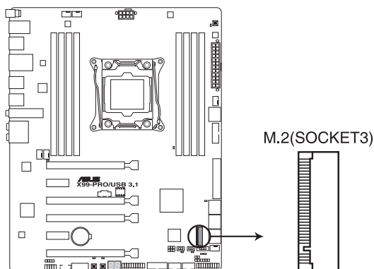
Connecteur M.2 de la X99-PRO / USB 3.1
