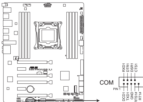
Connecteur pour port COM de la X99-PRO / USB 3.1
