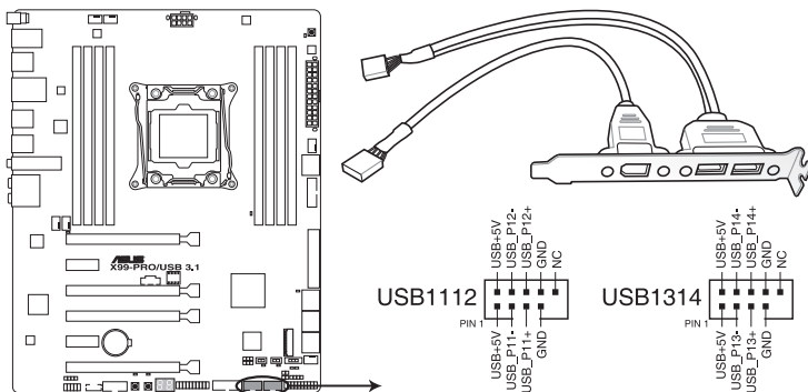
Connecteurs USB 2.0 de la X99-PRO / USB 3.1
