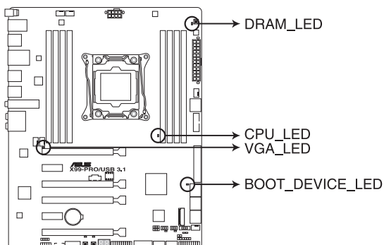
Témoins du POST de la X99-PRO / USB 3.1
