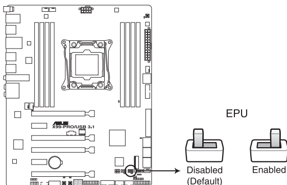
Interrupteur EPU de la X99-PRO / USB 3.1
