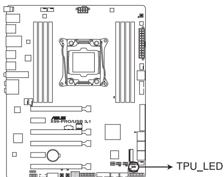
LED TPU de la X99-PRO / USB 3.1
