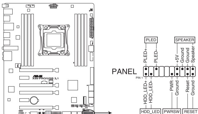
Connecteur panneau système de la X99-PRO / USB 3.1
