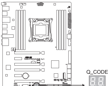
Témoins de débogage de la X99-PRO / USB 3.1
