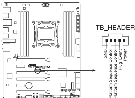
Connecteur Thunderbolt de la X99-PRO / USB 3.1
