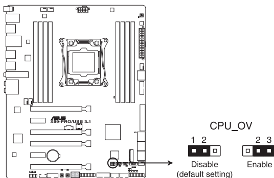
Jumper de surtension du processeur de la X99-PRO / USB 3.1
