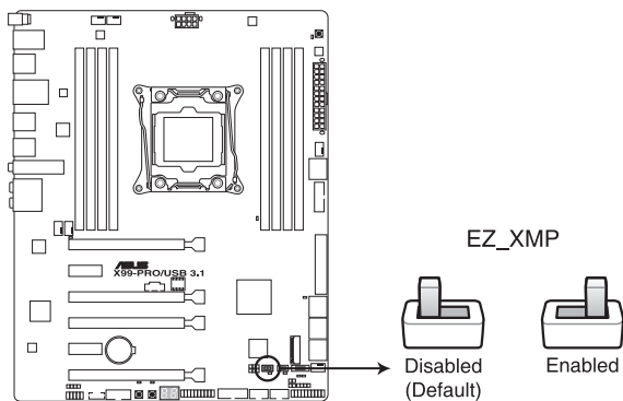
Interrupteur EZ XMP de la X99-PRO / USB 3.1
