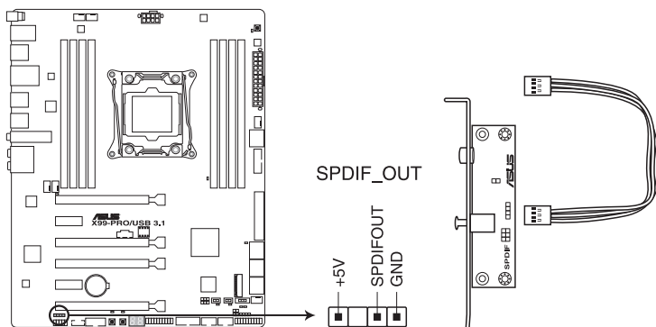
Connecteur audio numérique de la X99-PRO / USB 3.1
