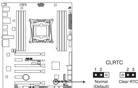
Jumper d'effacement de la mémoire CMOS de la X99-PRO / USB 3.1
