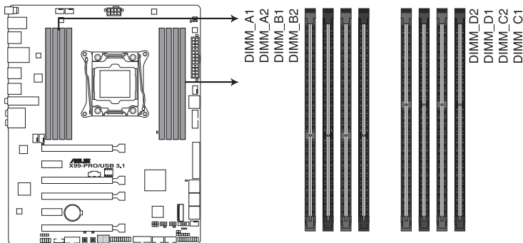
Interfaces de connexion pour modules mémoire DDR4 de la X99-PRO / USB 3.1
