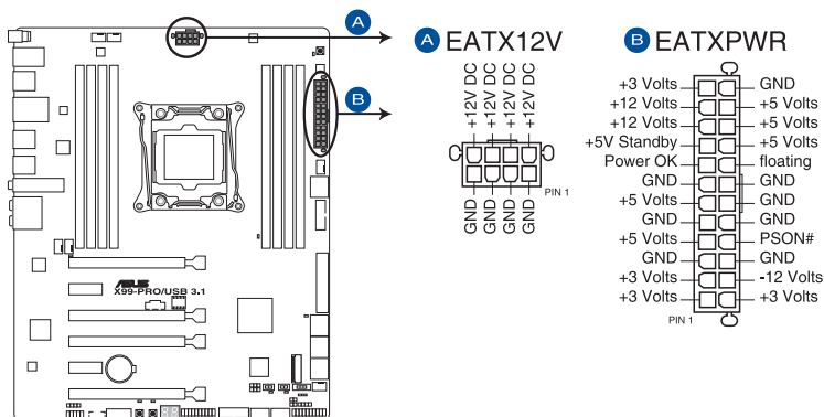
Connecteurs d'alimentation de la X99-PRO / USB 3.1
