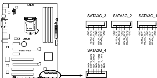
Connecteurs SATA 3Gb/s de la P8Z77-V LX
