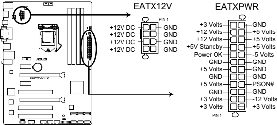
Connecteurs d'alimentation de la P8Z77-V LX
