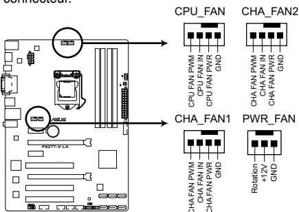
Connecteurs de ventilation de la P8Z77-V LX
