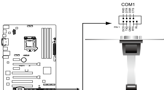
Connecteur pour port COM de la P8Z68-V LE
