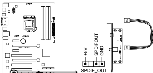
Connecteur audio numérique de la P8Z77-V LX
