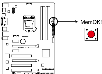
Interrupteur MemOK! de la P8Z77-V LX
