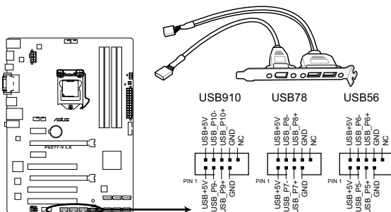
Connecteurs USB 2.0 de la P8Z77-V LX
