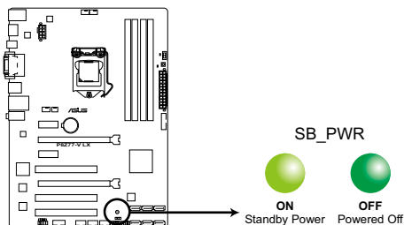
LED d'alimentation de la P8Z77-V LX
