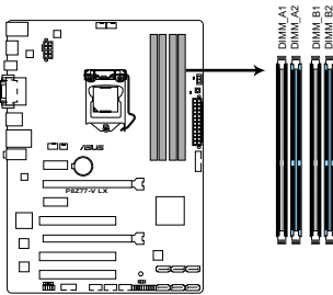
Slots DDR3 de la P8Z77-V LX
