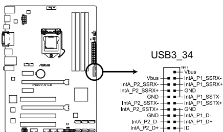
Connecteur USB 3.0 de la P8Z77-V LX
