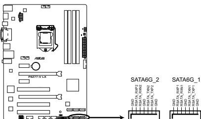
Connecteurs SATA 6.0Gbs de la P8Z77-V LX
