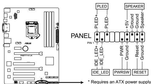
Connecteur panneau système de la P8Z77-V LX
