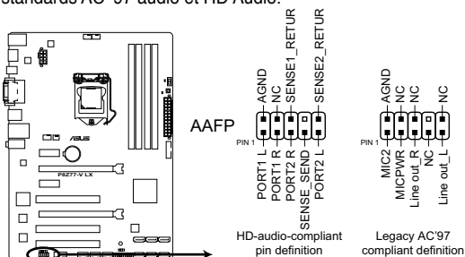
Connecteur audio pour panneau avant de la P8Z77-V LX
