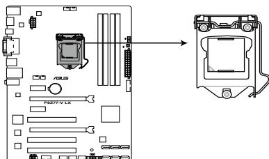
Socket 1155 de la P8Z77-V LX
