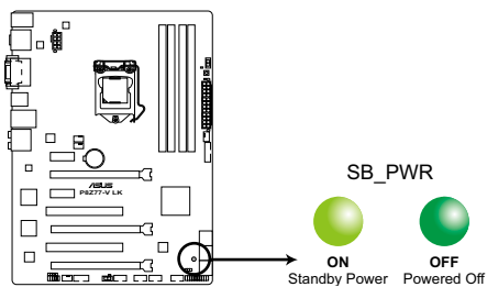
LED d'alimentation de la P8Z77-V LK
