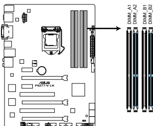
Interfaces de connexion DDR3 de la P8Z77-V LK
