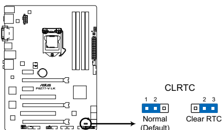
Jumper d'effacement de la mémoire CMOS de la P8Z77-V LK
