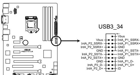
Connecteur USB 3.0 de la P8Z77-V LK
