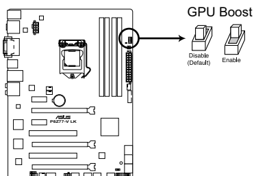
Interrupteur GPU Boost de la P8Z77-V LK
