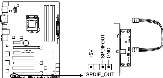
Connecteur audio numérique de la P8Z77-V LK
