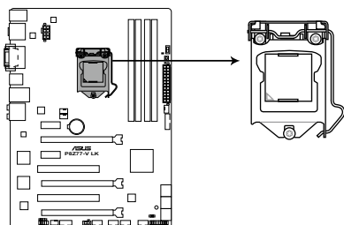
Interface de connexion 1155 de la P8Z77-V LK
