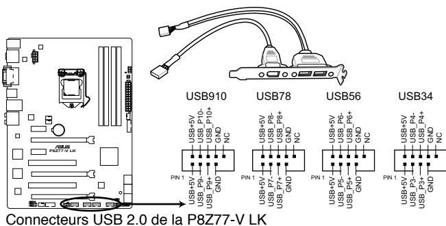
Connecteurs USB 2.0 de la P8277-V LK
