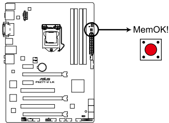
Interrupteur MemOK! de la P8Z77-V LK
