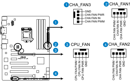
Connecteurs de ventilation de la P8Z77-V LK
