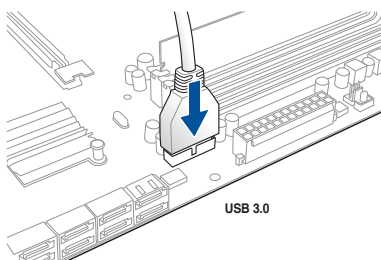
Connecteur USB 3.0
