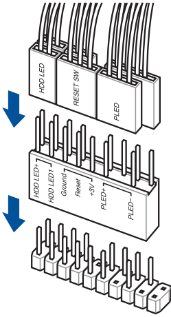
安装 USB 2.0 连接插槽
