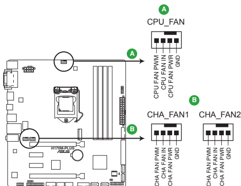
H170M-PLUS Fan connectors
