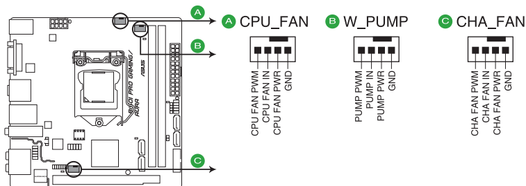
B150I PRO GAMING/AURA Fan connectors
