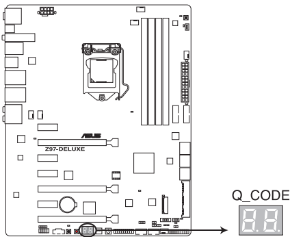
Témoins de débogage de la Z97-DELUXE
