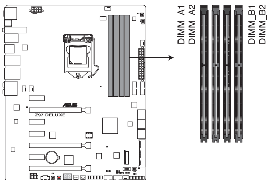
Interfaces de connexion pour modules mémoire DDR3 de la Z97-DELUXE
