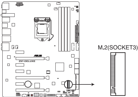
Connecteur M.2 de la Z97-DELUXE
