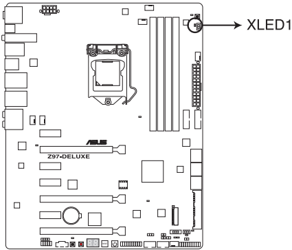
Témoin EZ XMP de la Z97-DELUXE
