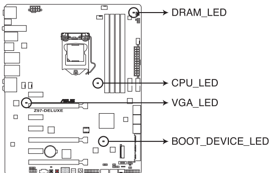
Témoin du POST de la Z97-DELUXE
