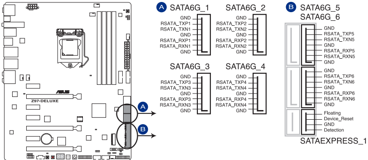
Connecteurs SATA 6.0Gbs de la Z97-DELUXE
