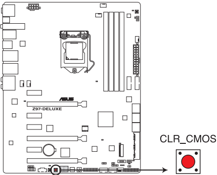
Bouton d'effacement de la mémoire CMOS de la Z97-DELUXE
