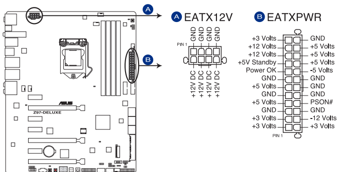
Connecteurs d'alimentation de la Z97-DELUXE
