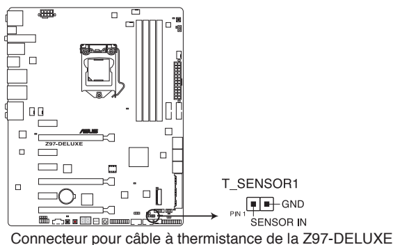
Connecteur pour câble à thermistance de la Z97-DELUXE
