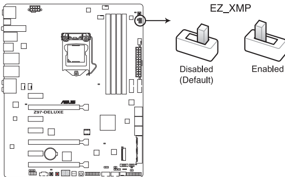
Interrupteur EZ XMP de la Z97-DELUXE
