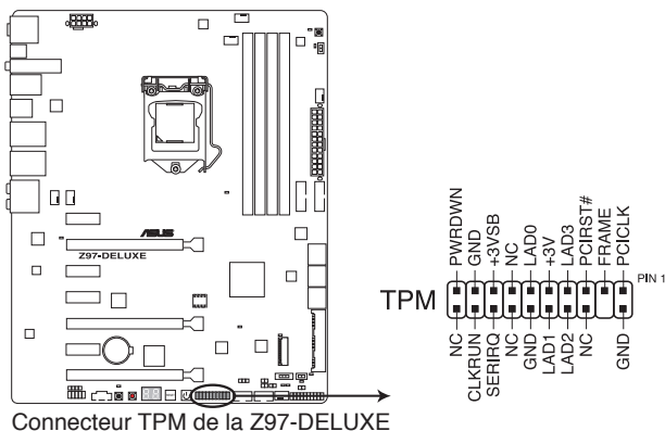
Connecteur TPM de la Z97-DELUXE
