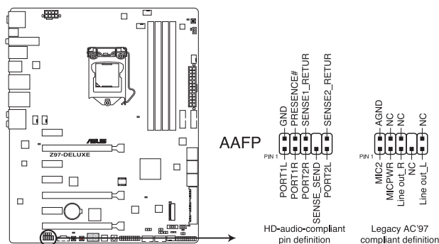
Connecteur audio pour panneau avant de la Z97-DELUXE
