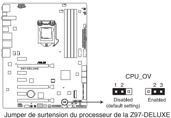
Jumper de surtension du processeur de la Z97-DELUXE
