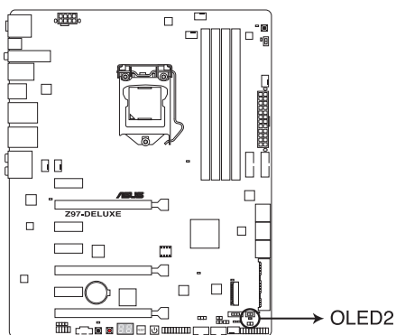
Témoin EPU de la Z97-DELUXE
