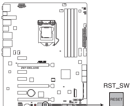
Bouton de réinitialisation de la Z97-DELUXE
