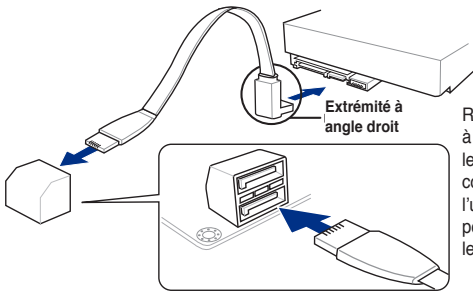
Connecteurs SATA 6.0Gbs de la Z97-DELUXE
