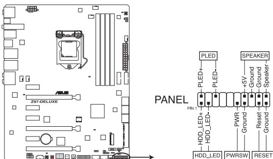
Connecteur panneau système de la Z97-DELUXE
