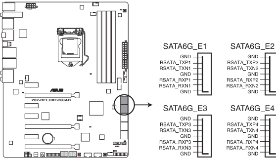
Connecteurs SATA 6Gb/s Marvell de la Z97-DELUXE
