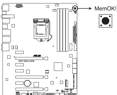
Bouton MemOK! de la Z97-DELUXE
