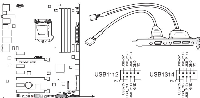
Connecteurs USB 2.0 de la Z97-DELUXE
