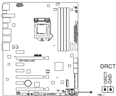
Connecteur DirectKey de la Z97-DELUXE
