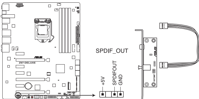
Connecteur audio numérique de la Z97-DELUXE
