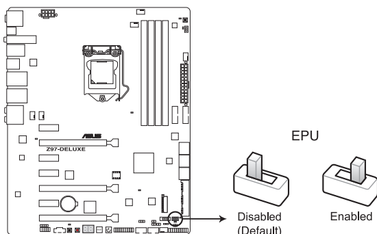
Interrupteur EPU de la Z97-DELUXE
