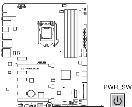
Bouton de mise sous tension de la Z97-DELUXE
