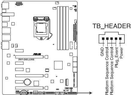
Connecteur Thunderbolt de la Z97-DELUXE
