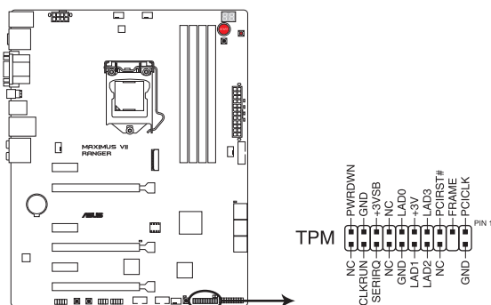
Connecteur TPM de la MAXIMUS VII RANGER
