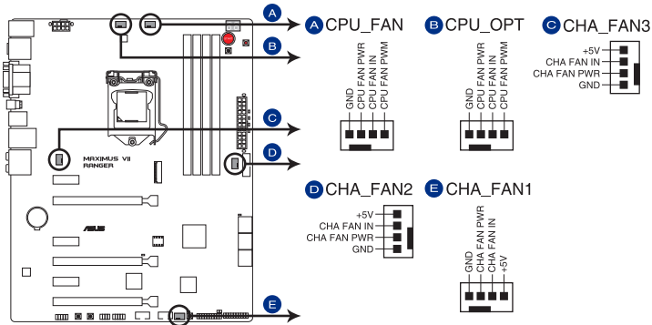
Connecteurs de ventilation de la MAXIMUS VII RANGER
