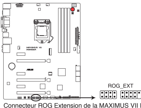
Connecteur ROG Extension de la MAXIMUS VII RANGER
