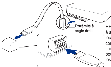
Connecteurs SATA 6.0Gbs de la MAXIMUS VII RANGER
