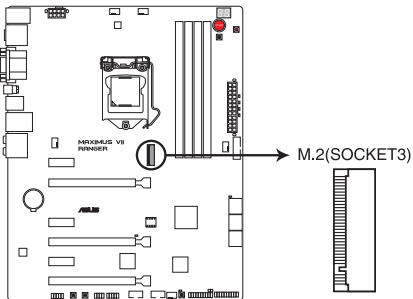
Connecteur M.2 de la MAXIMUS VII RANGER
