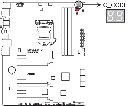
Témoins de débogage de la MAXIMUS VII RANGER
