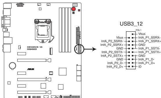
Connecteur USB 3.0 de la MAXIMUS VII RANGER
