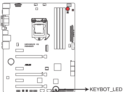
Témoin KeyBot de la MAXIMUS VII RANGER
