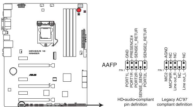
Connecteur audio pour panneau avant de la MAXIMUS VII RANGER
