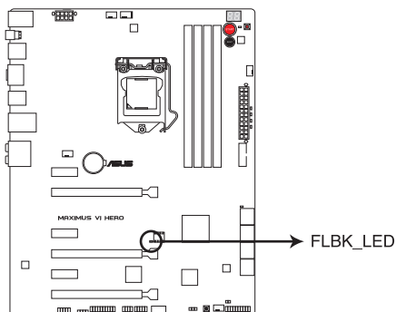
Témoin USB BIOS Flashback de la MAXIMUS VII RANGER
