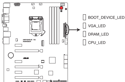
Témoins Q-LED de la MAXIMUS VII RANGER
