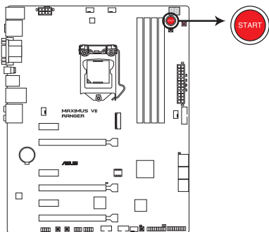
Bouton de mise sous tension de la MAXIMUS VII RANGER
