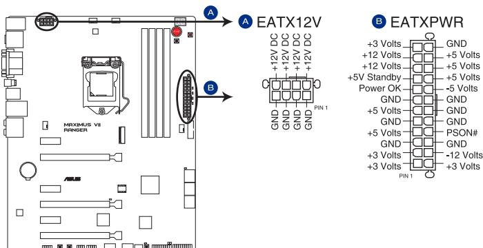
Connecteurs d'alimentation de la MAXIMUS VII RANGER
