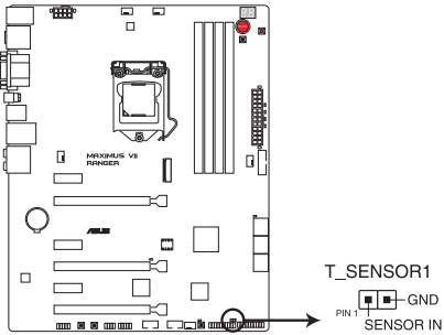
Connecteur pour câble à thermistance de la MAXIMUS VII RANGER
