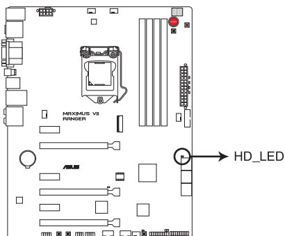
Témoin d'activité de disque dur de la MAXIMUS VII RANGER
