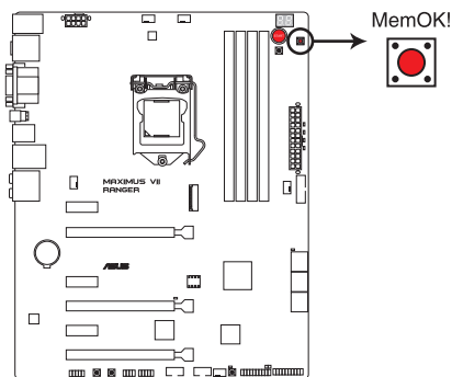
Bouton MemOK! de la MAXIMUS VII RANGER
