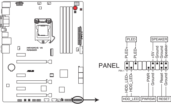
Connecteur panneau système de la MAXIMUS VII RANGER
