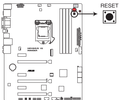
Bouton de réinitialisation de la MAXIMUS VII RANGER
