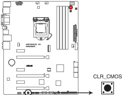
Bouton d'effacement de la mémoire CMOS de la MAXIMUS VII RANGER
