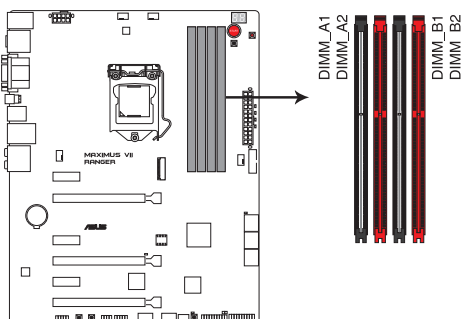
Interfaces de connexion pour modules mémoire DDR3 de la MAXIMUS VII RANGER
