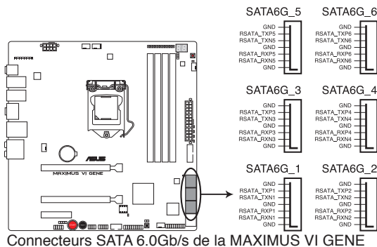
Connecteurs SATA 6.0Gb/s de la MAXIMUS VI GENE
