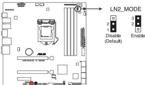
Jumper LN2 de la MAXIMUS VI GENE
