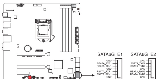
Connecteurs SATA 6Gb/s de la MAXIMUS VI GENE
