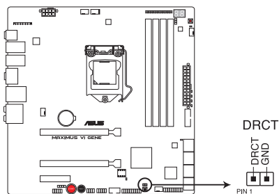
Connecteur DirectKey de la MAXIMUS VI GENE
