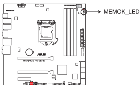
Témoin d'activité MemOK! de la MAXIMUS VI GENE
