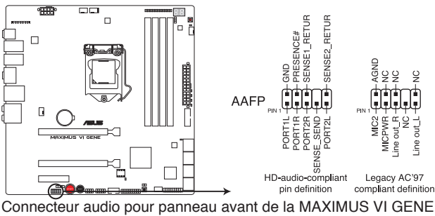
Connecteur audio pour panneau avant de la MAXIMUS VI GENE
