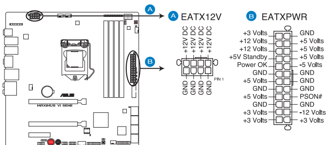
Connecteurs d'alimentation de la MAXIMUS VI GENE
