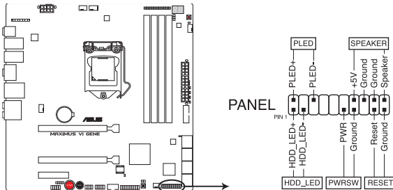
Connecteur panneau système de la MAXIMUS VI GENE
