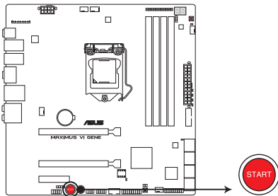
Témoin d'alimentation de la MAXIMUS VI GENE
