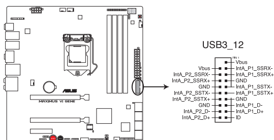
Connecteur USB 3.0 de la MAXIMUS VI GENE
