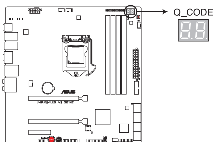
Témoins de débogage de la MAXIMUS VI GENE
