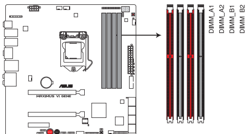
Interfaces de connexion pour modules mémoire DDR3 de la MAXIMUS VI GENE
