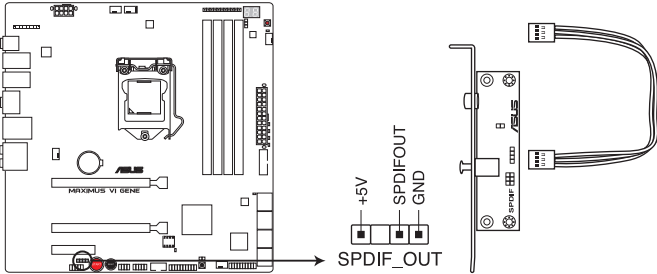
Connecteur audio numérique de la MAXIMUS VI GENE
