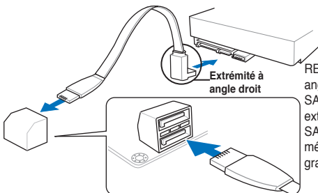
Connecteurs SATA 6.0Gb/s de la MAXIMUS VI GENE
