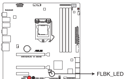
LED USB BIOS Flashback de la MAXIMUS VI GENE
