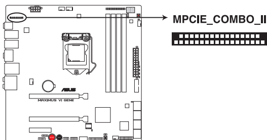
Connecteur M.2 (NGFF) de la MAXIMUS VI GENE
