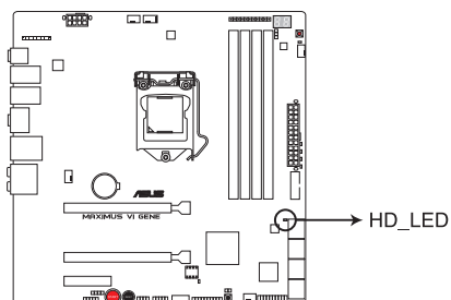
Témoin d'activité de disque dur de la MAXIMUS VI GENE
