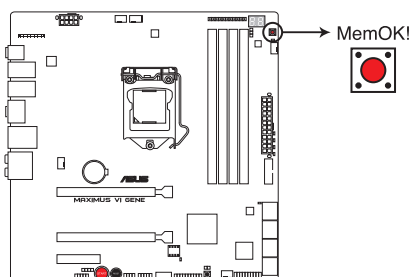
Bouton MemOK! de la MAXIMUS VI GENE
