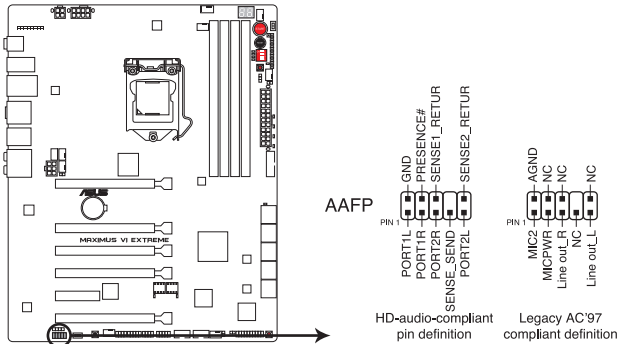
Connecteur audio pour panneau avant de la MAXIMUS VI EXTREME
