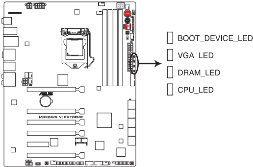
Témoins Q-LED de la MAXIMUS VI EXTREME
