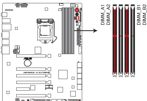
Interfaces de connexion pour modules mémoire DDR3 de la MAXIMUS VI EXTREME
