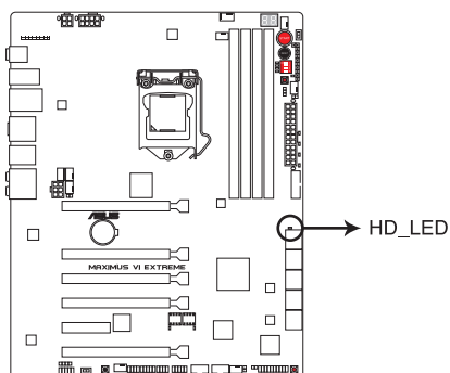
Témoin d'activité de disque dur de la MAXIMUS VI EXTREME
