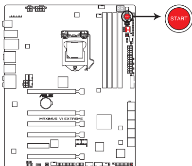
Bouton de mise sous tension de la MAXIMUS VI EXTREME
