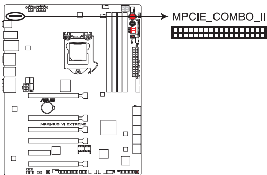
Connecteur M.2 (NGFF) de la MAXIMUS VI EXTREME
