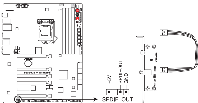
Connecteur audio numérique de la MAXIMUS VI EXTREME
