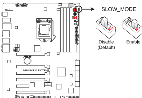
Interrupteur Slow Mode de la MAXIMUS VI EXTREME
