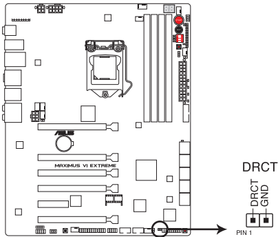
Connecteur DirectKey de la MAXIMUS VI EXTREME
