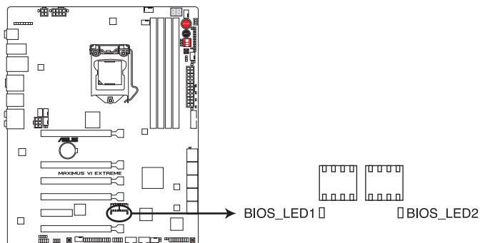
LED BIOS de la MAXIMUS VI EXTREME
