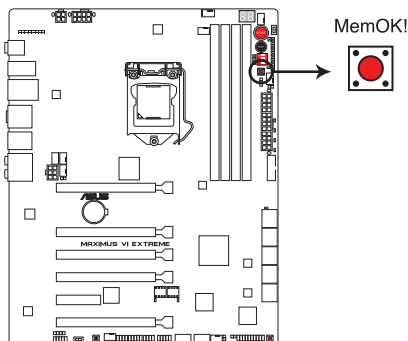
Bouton MemOK! de la MAXIMUS VI EXTREME
