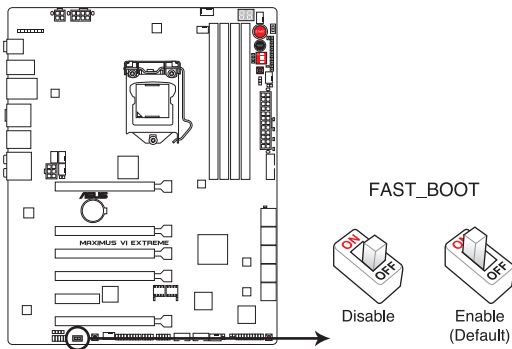
Interrupteur FastBoot de la MAXIMUS VI EXTREME
