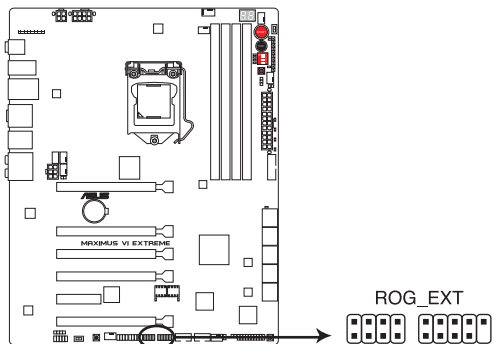
Connecteur ROG Extension de la MAXIMUS VI EXTREME
