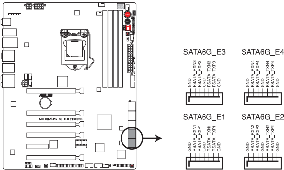
Connecteurs SATA 6Gb/s de la MAXIMUS VI EXTREME
