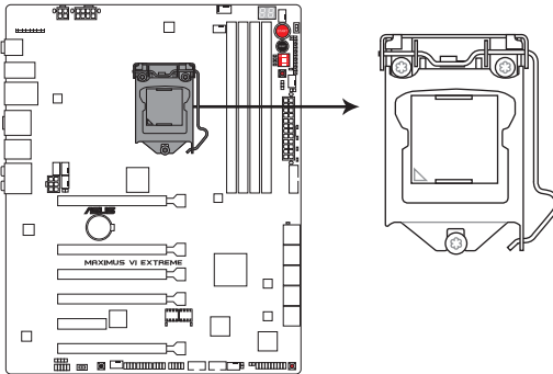
Interface de connexion LGA1150 de la MAXIMUS VI EXTREME
