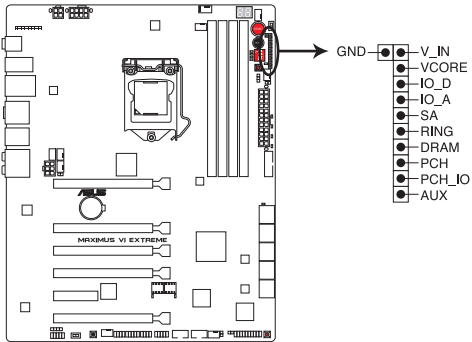
Zone Probelt de la MAXIMUS VI EXTREME
