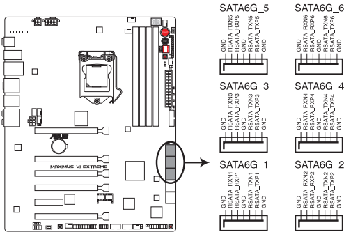
Connecteurs SATA 6.0Gb/s de la MAXIMUS VI EXTREME
