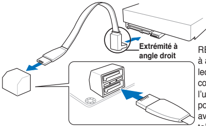
Connecteurs SATA 6.0Gb/s de la MAXIMUS VI EXTREME
