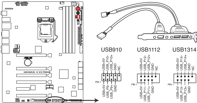
Connecteurs USB 2.0 de la MAXIMUS VI EXTREME
