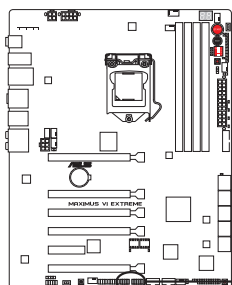
Connecteur ROG_EXT de la MAXIMUS VI EXTREME
