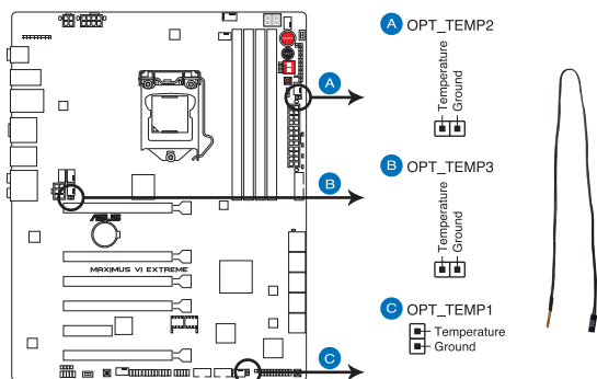
Connecteurs pour capteurs thermique de la MAXIMUS VI EXTREME
