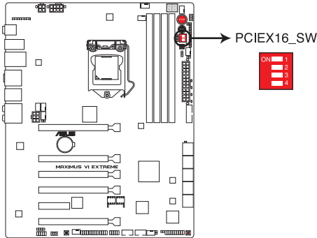
Interrupteur de voie PCIe x16 de la MAXIMUS VI EXTREME
