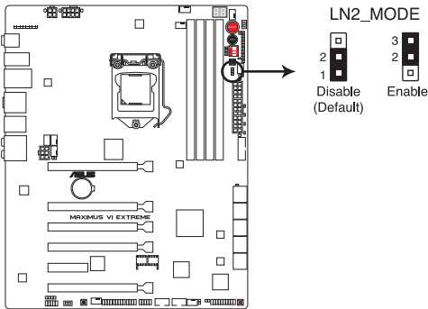
Jumper LN2 de la MAXIMUS VI EXTREME
