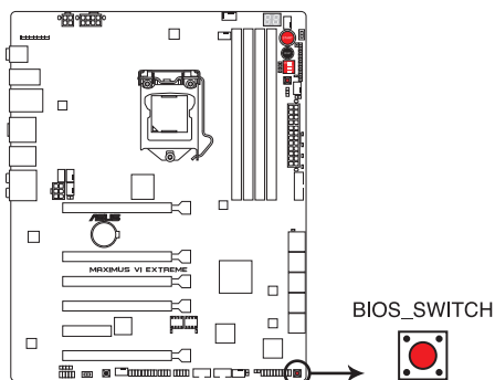
Bouton de sélection du BIOS de la MAXIMUS VI EXTREME
