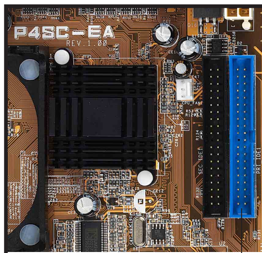
第一組 IDE 排線插座 (PRI IDE1)
